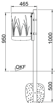
7039-65 Seitenansicht Pfostenbefestigung
