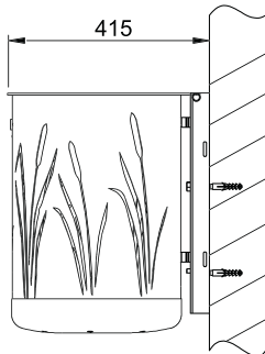
7039-65 Seitenansicht Wandbefestigung
